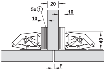
Montaje intermedio/gemelo
