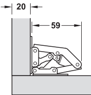
Montaje angular
