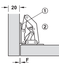
Montaje enrasado
