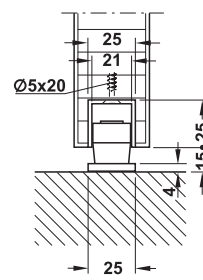
Rodillo de la guía para suelo, montaje sobrepuesto
