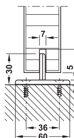
Guía para suelo en forma de T
