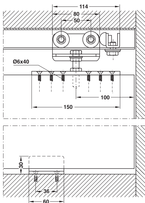
Corte carro de rodillos y guía de suelo en forma de T
