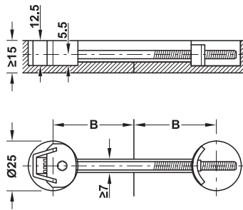
Patrón de perforación
